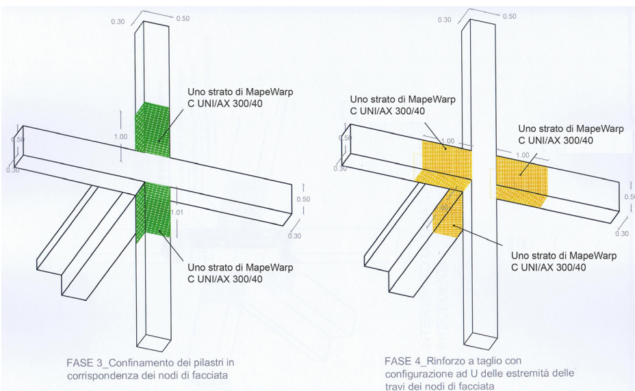
La grafica delle fasi di intervento sui diversi nodi trave-pilastro.
