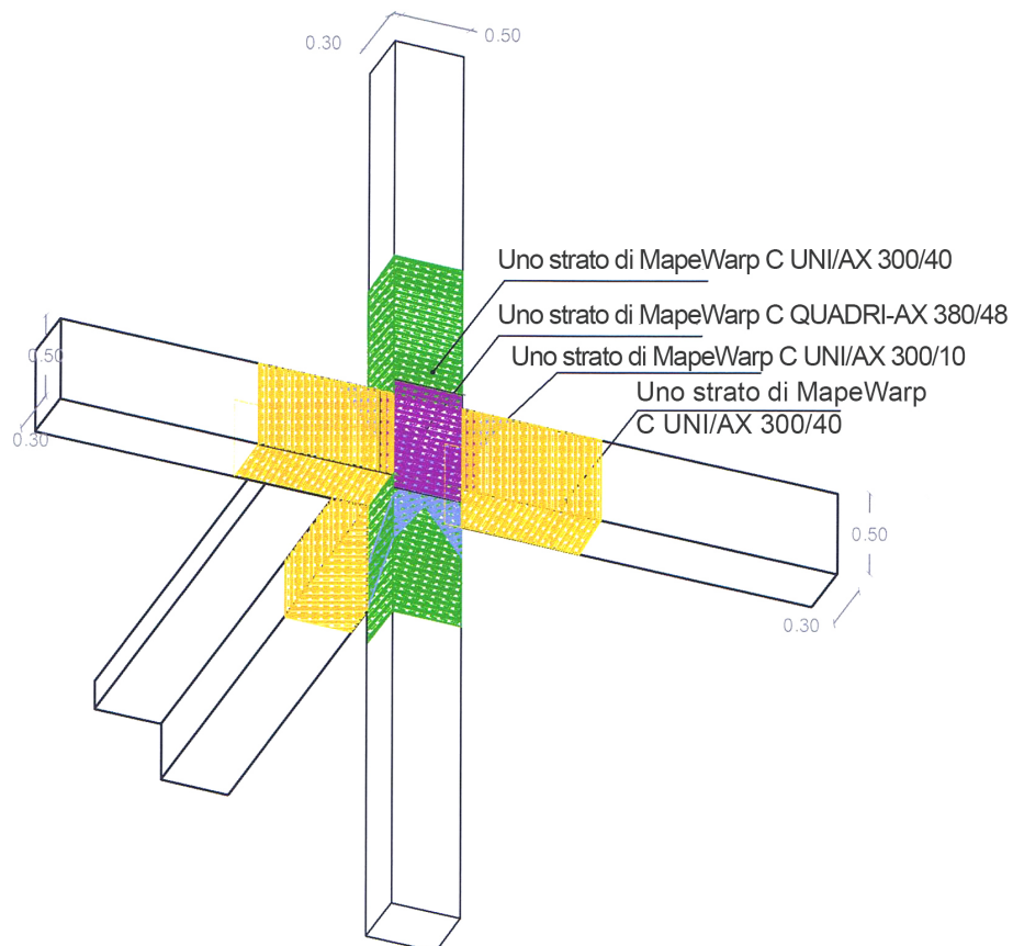
Sovrapposizione grafica degli interventi effettuati sui nodi trave-pilastro nel condominio "Gemma 84".
