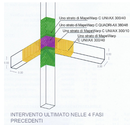
La grafica delle fasi di intervento sui diversi nodi trave-pilastro.
